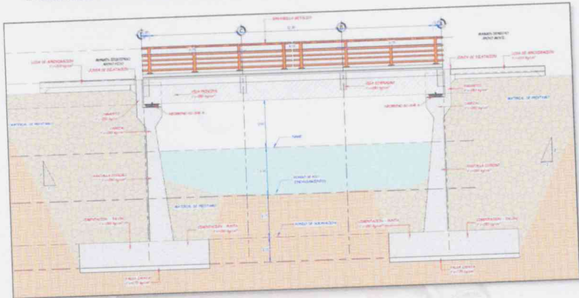
Figura. Sección de Planteamiento Principal.
