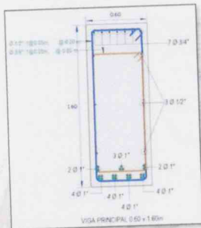
Secciones de viga corte A-A
